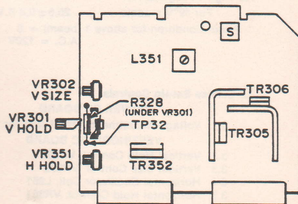
FIGURE 2 VERT./HORIZ. BOARD
